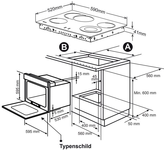
Abbildung 10 - Bündige Ofeninstallation
