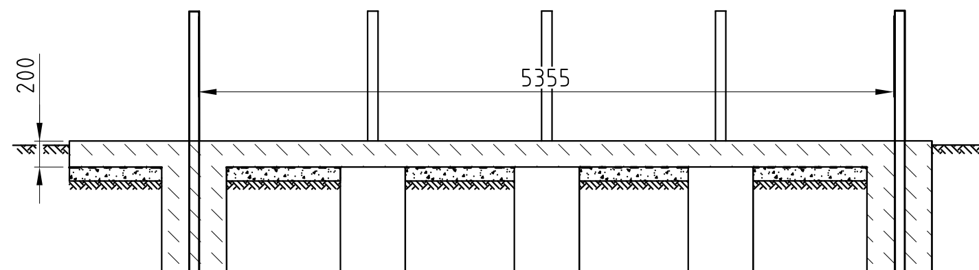
Schnitt B-B
