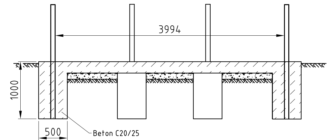
Schnitt A-A
