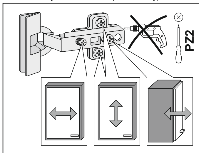
Türverstellungsschema (falls erforderlich) Door adjustment scheme (if necessary)
