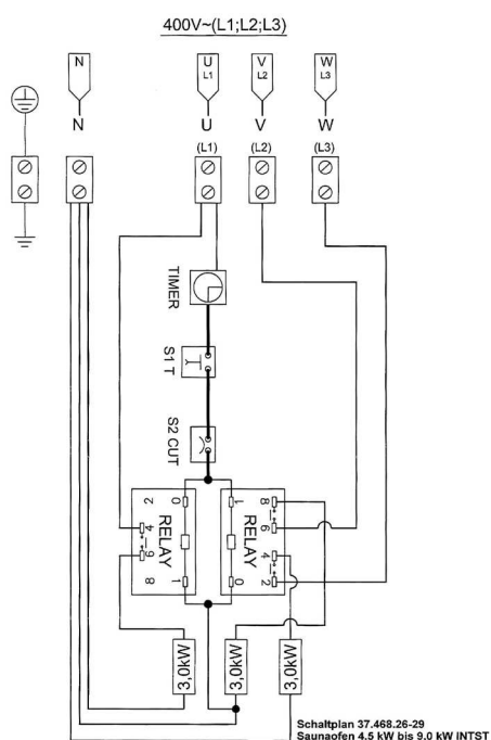
Sistema de mando interior de la estufa de sauna 9 kW
