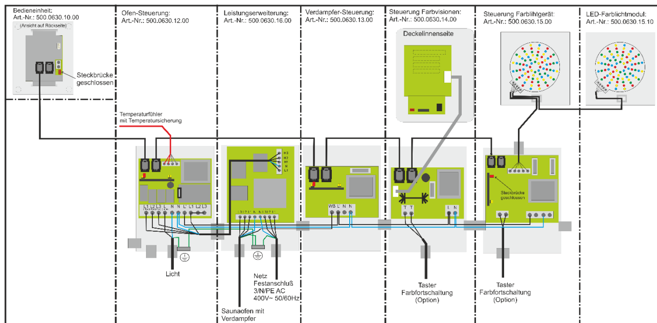
Abbildung 4 Anschlussbeispiel Ofensteuerung
