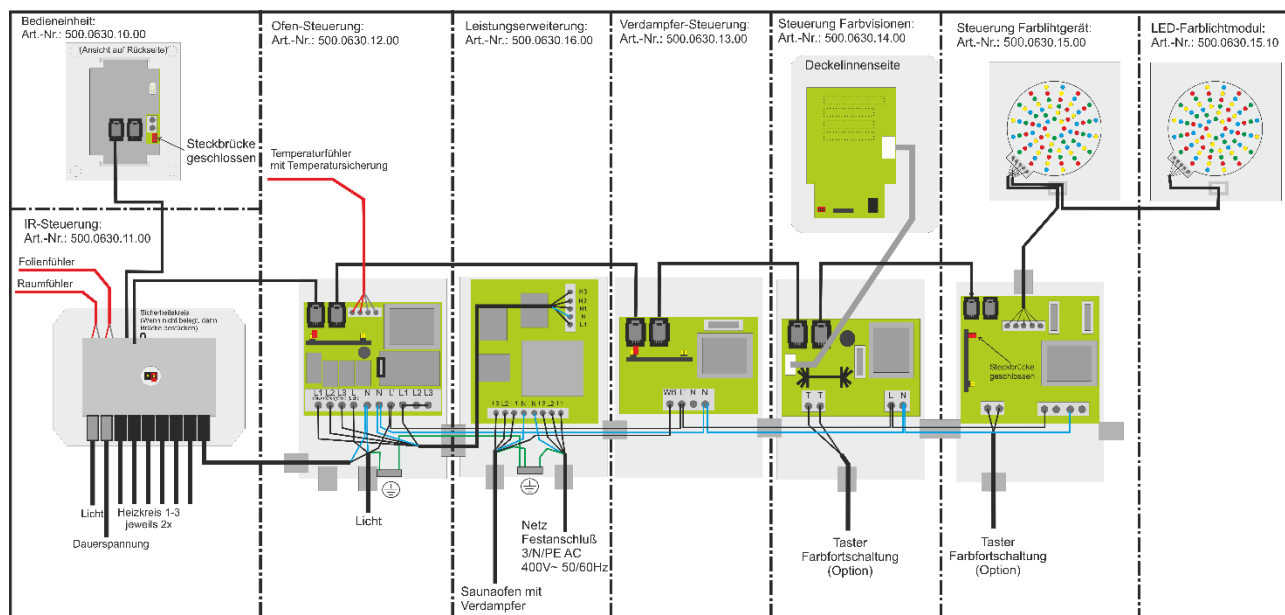
Abbildung 5 Anschlussbeispiel Kombisteuerung
