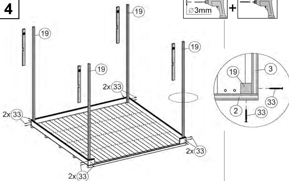
Abbildung Art.-Nr.: 227.2121.10400
