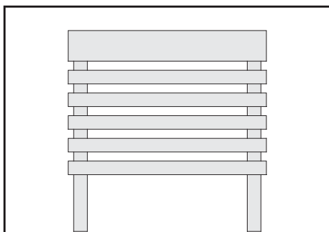
2 x Q1 | 474 x 590 x 32 mm | ID 2252
