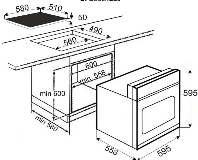
Einbauskizze
