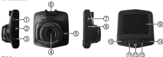
Bild 1: Kamera
