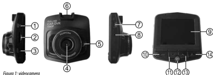
Figura 1: videocamera
