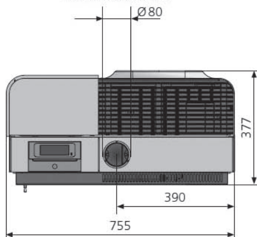
Rauchrohranschluss
