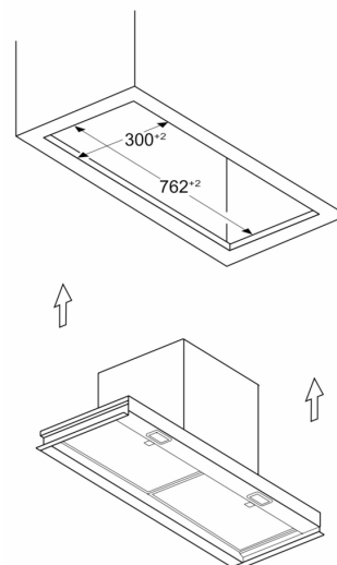
Maße in mm Einbaubeispiel in Möbelausschnitt
