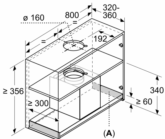
Maße in mm Einbaubeispiel
