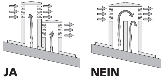
Abb. 5. Eigenschaften des Schornsteins
