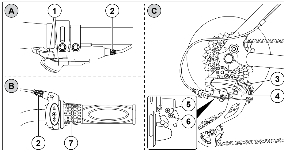
Abb. 61 Kettenschaltung hinten
