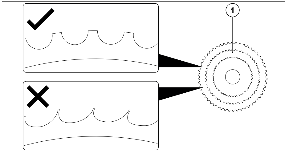
Abb. 54 Zahnkranzverschleiß
