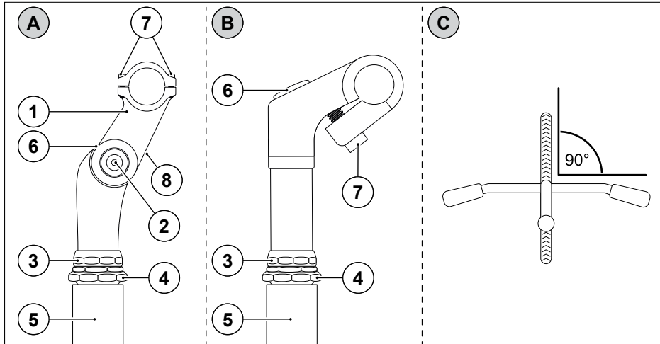
Abb. 46 Lenker einstellen
