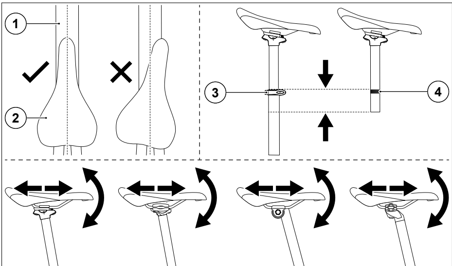
Abb. 40 Sattel und Sattelstütze
