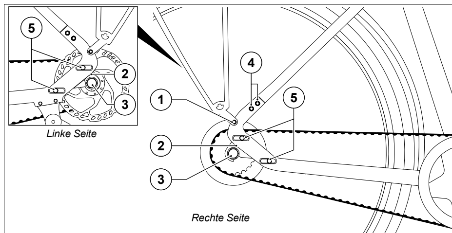
Abb. 57 Riemen wechseln
