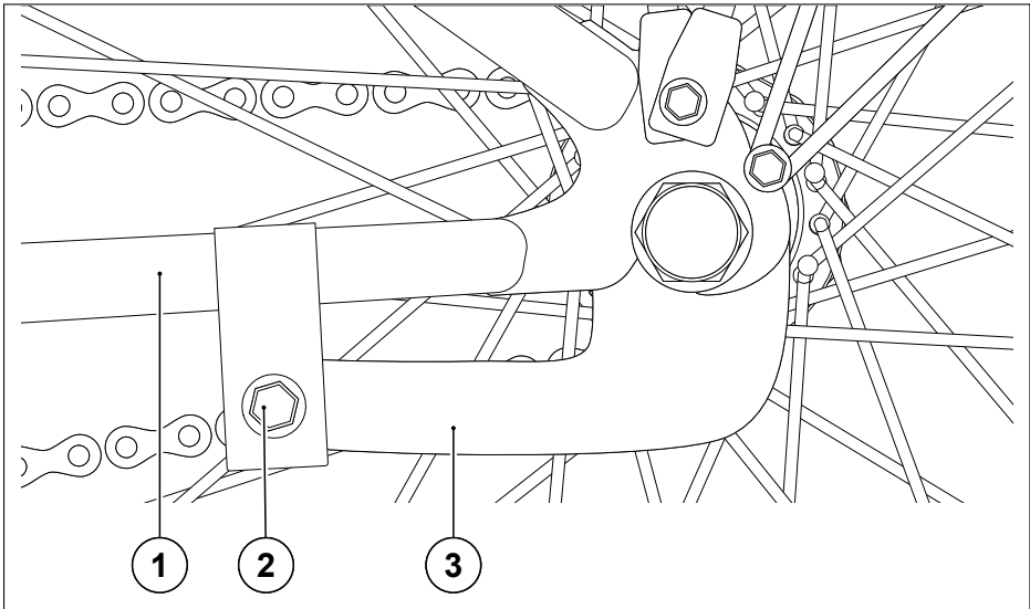
Abb. 37 Rücktrittbremse
