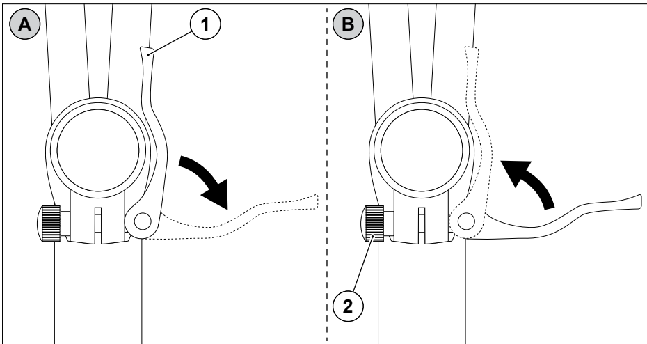
Abb. 47 Schnellspanner
