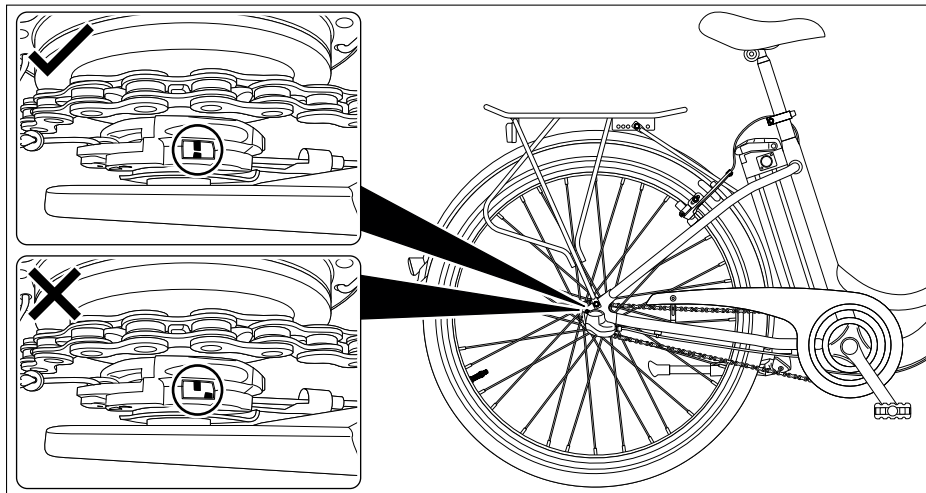
Abb. 62 Einstellung Nabenschaltung
