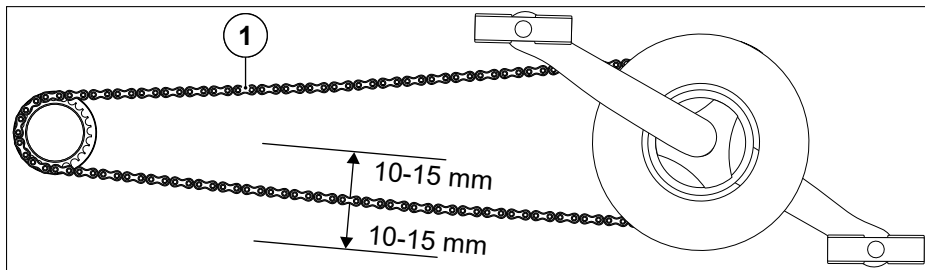
Abb. 55 Kettenspannung prüfen
