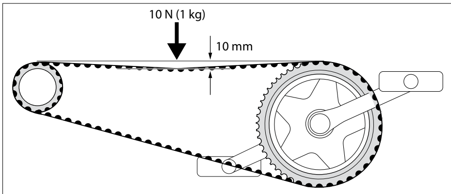
Abb. 59 Riemen ­ spannung prüfen (behelfsmäßig)
