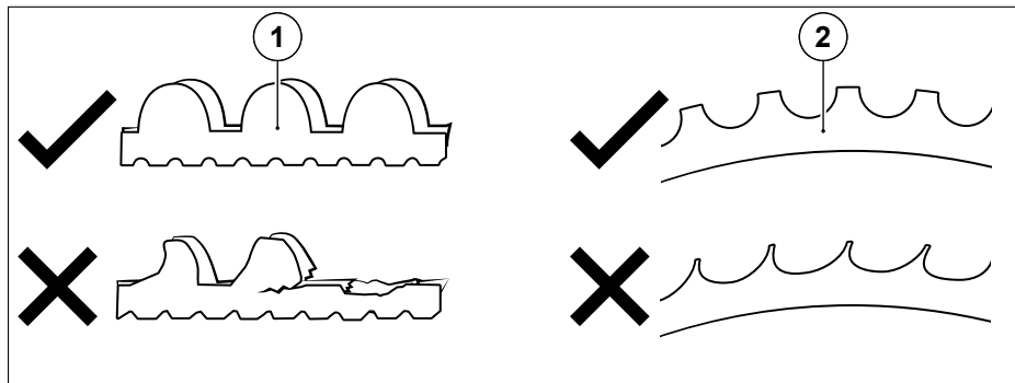
Abb. 56 Riemen- und Riemenscheibenverschleiß
