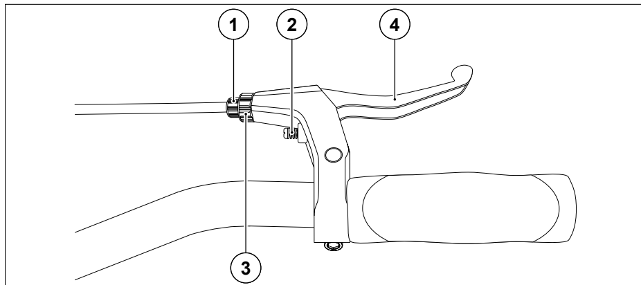
Abb. 34 Bremshebeleinstellung
