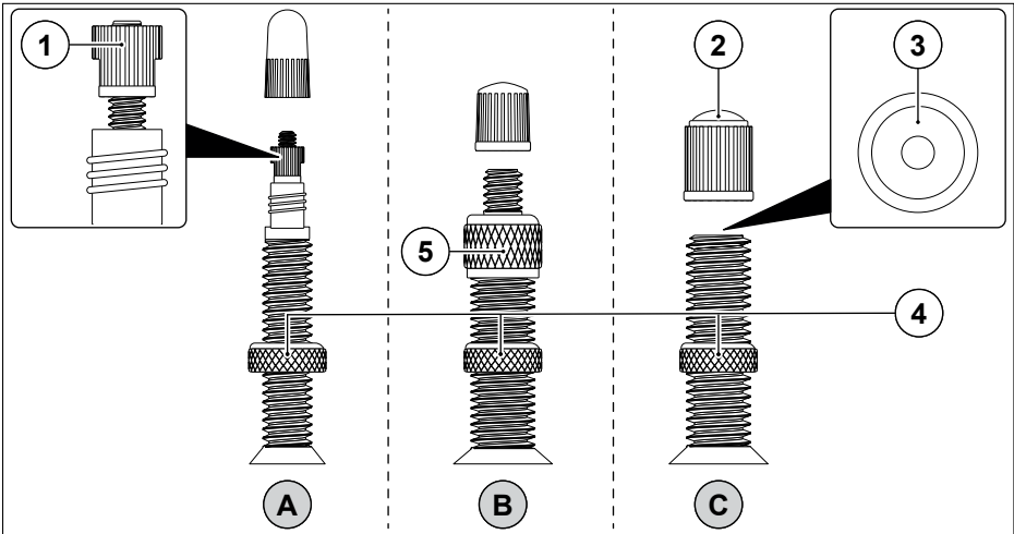
Abb. 39 Ventilvarianten
