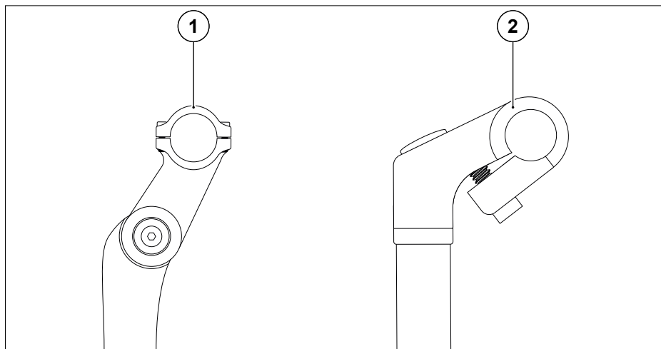
Abb. 43 Vorbauarten
