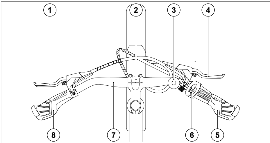
Abb. 42 Lenker und Vorbau
