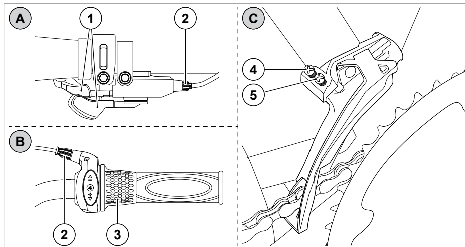
Abb. 60 Kettenschaltung vorne
