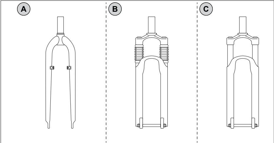
Abb. 25 Gabel-Typen
