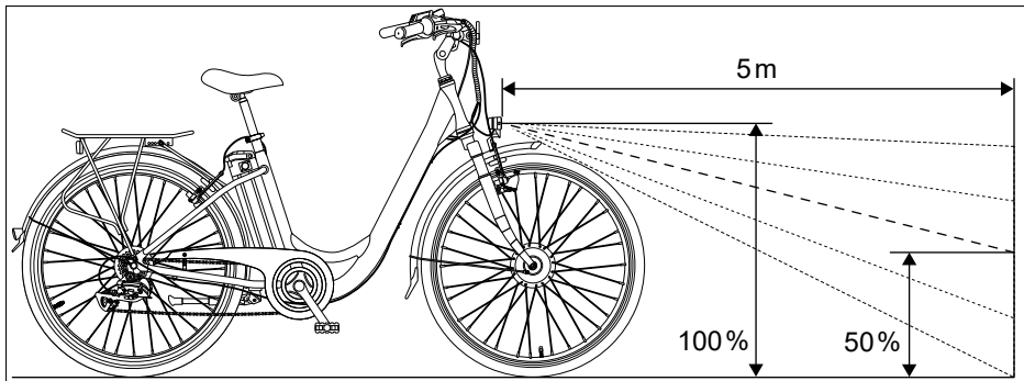
Abb. 49 Einstellung Beleuchtung
