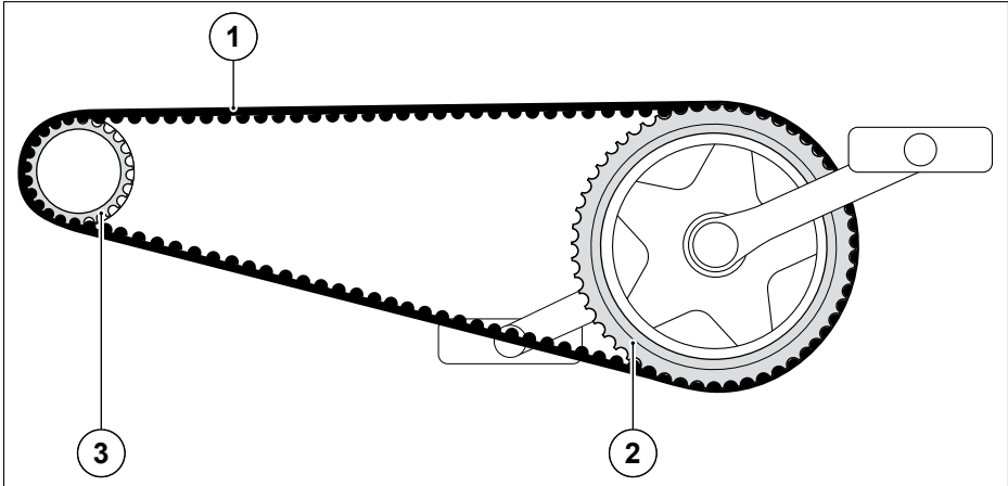
Abb. 28 Riemenantrieb
