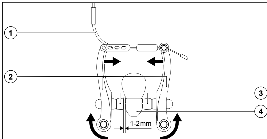
Abb. 36 Felgenbremse
