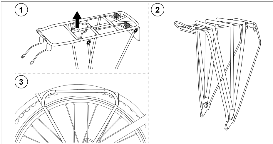
Abb. 50 Gepäckträgertypen
