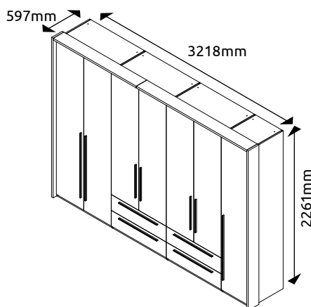
P74A/PN LWH - 3218x0597x2261
