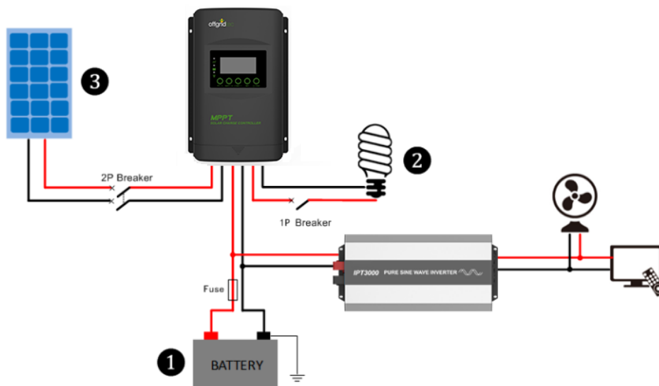
Abb. 2.2 Schaltplan
