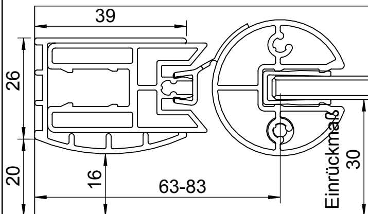
DETAIL A 1 : 1
