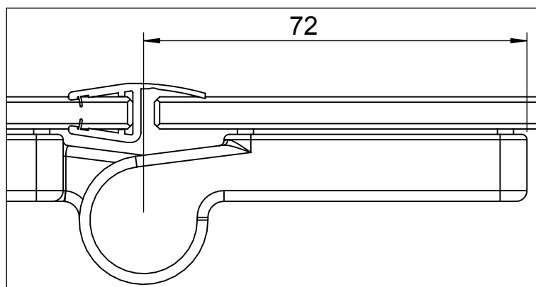
DETAIL B 1 : 1
