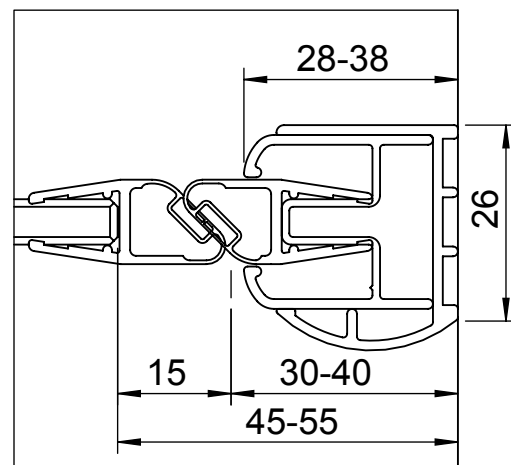
DETAIL C 1 : 1
