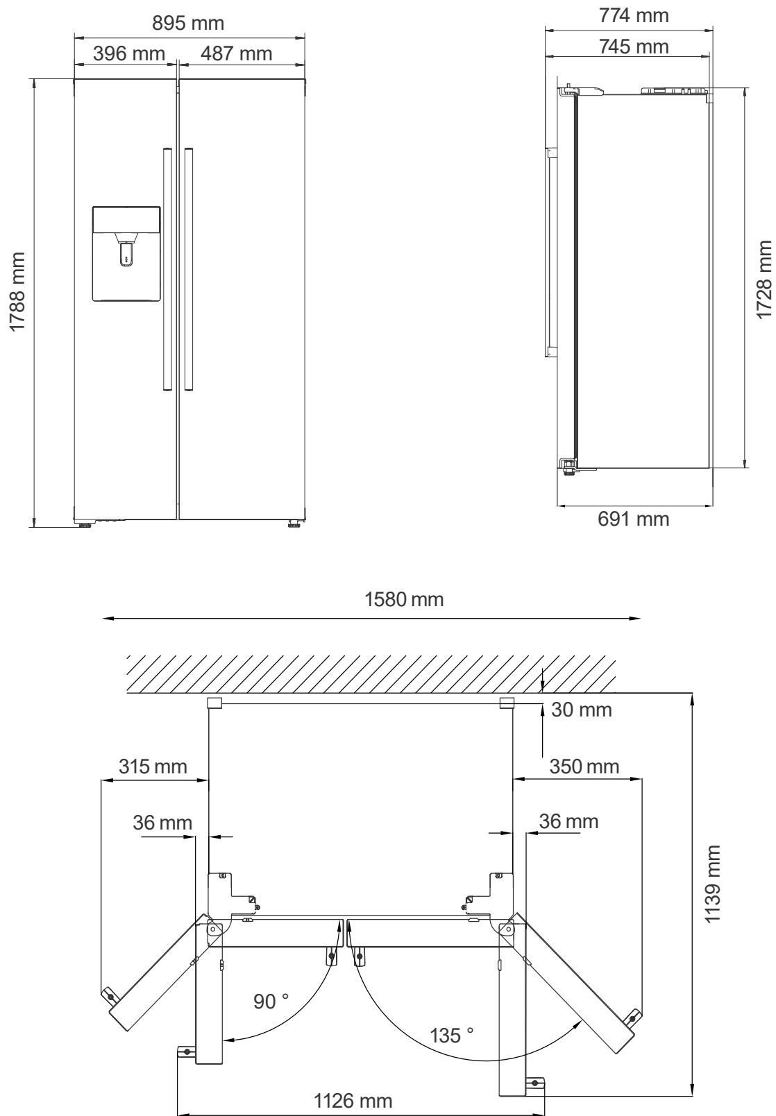
Grafik Raumbedarf (bei geschlossener und bei geöffneter Tür)
