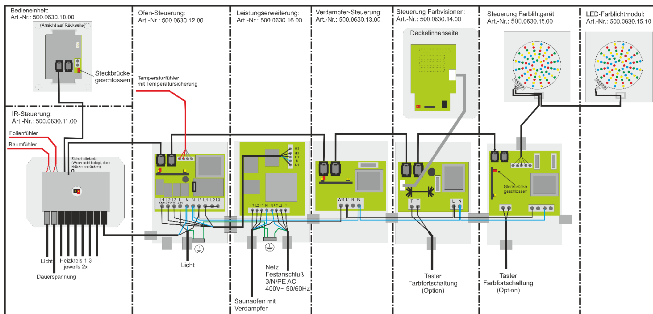
Abbildung 5 Anschlussbeispiel Kombisteuerung
