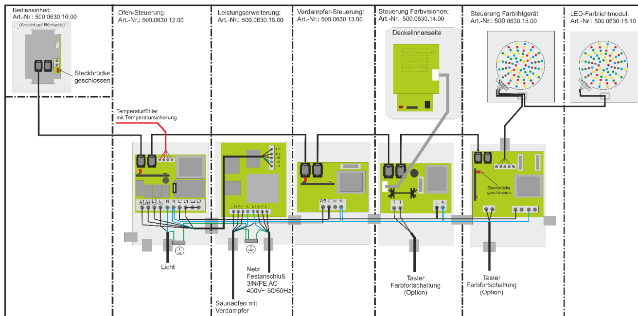
Abbildung 4 Anschlussbeispiel Ofensteuerung
