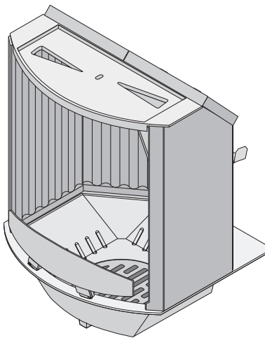
Abb. montierter Feuerraum
