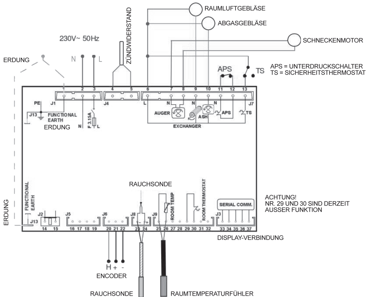
Abb. 15: Schaltplan der Platine
