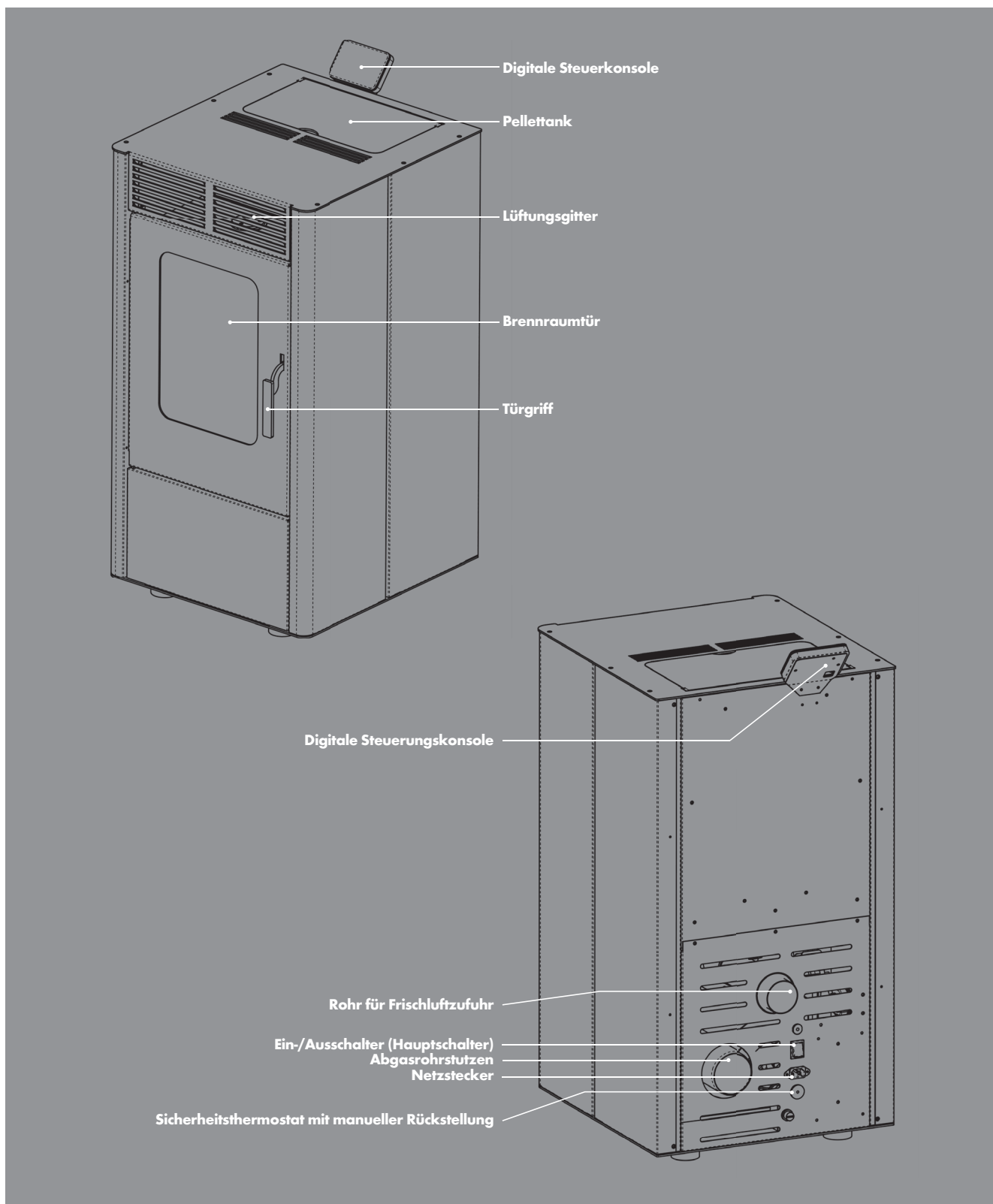
Abb. 1a: Geräteübersicht (Abbildung modellabhängig)
