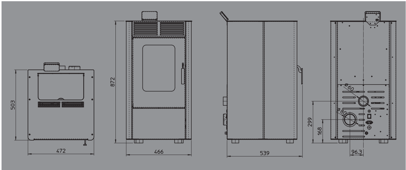
Abb. 1b: Geräteabmessungen (alle Maßangaben in mm)
