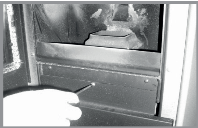
Abb. 13a: Öffnen der Frontplatte
