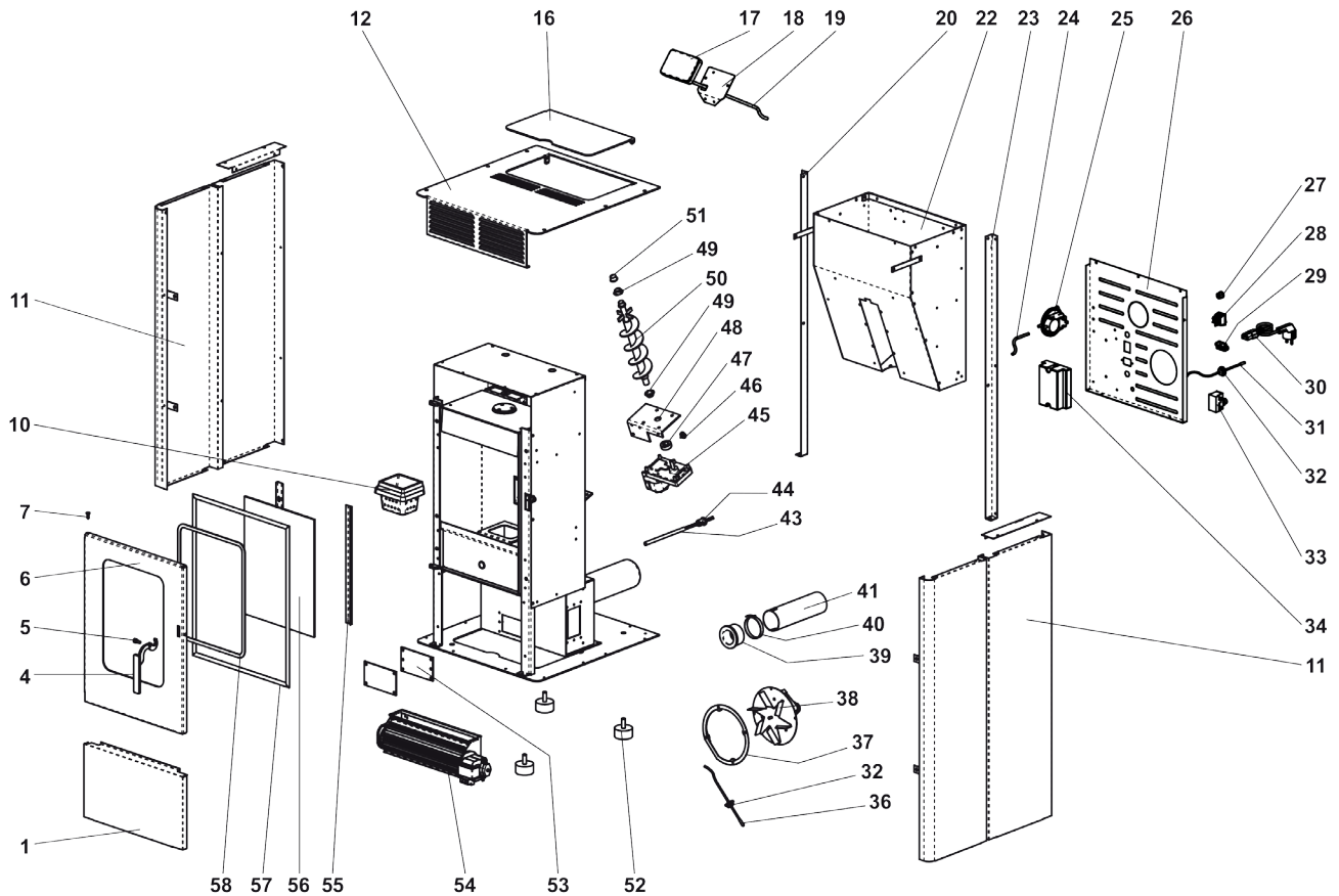
Abb. 14 Explosionszeichnung
