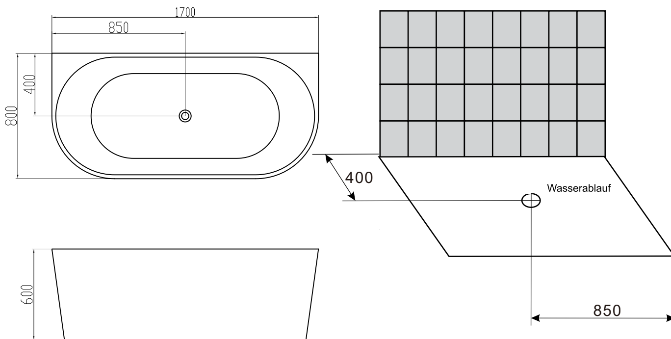
Maße Querschnitt
