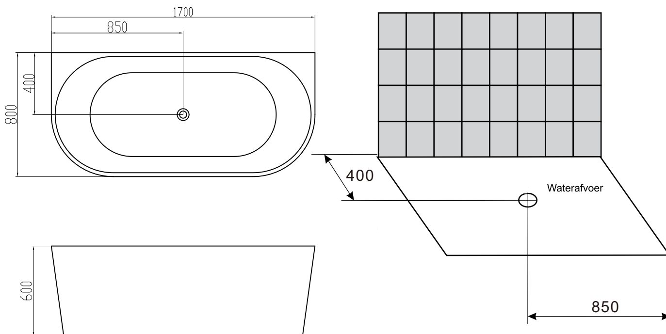
Afmetingen doorsnede
