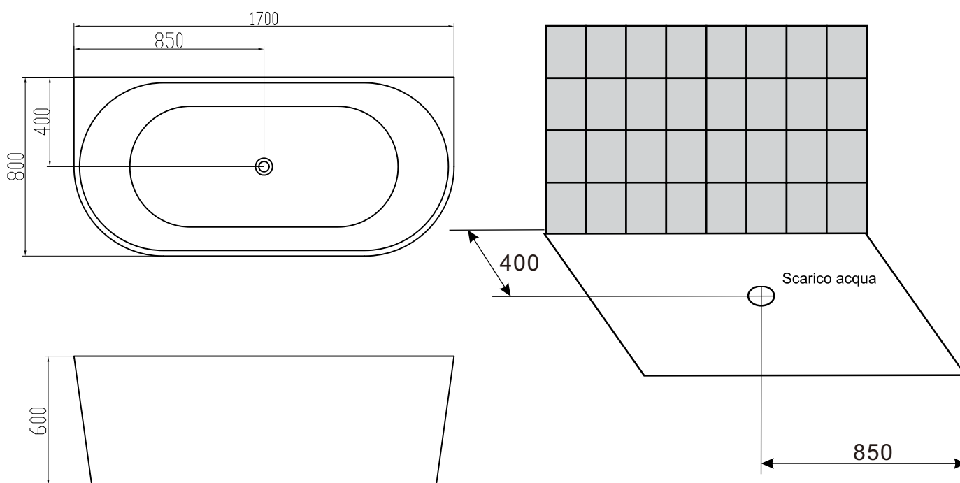
Dimensioni sezione
