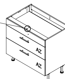
UC936-3D
