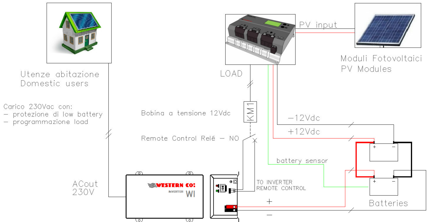
Fig. 3 Schema di collegamento WI800-12
