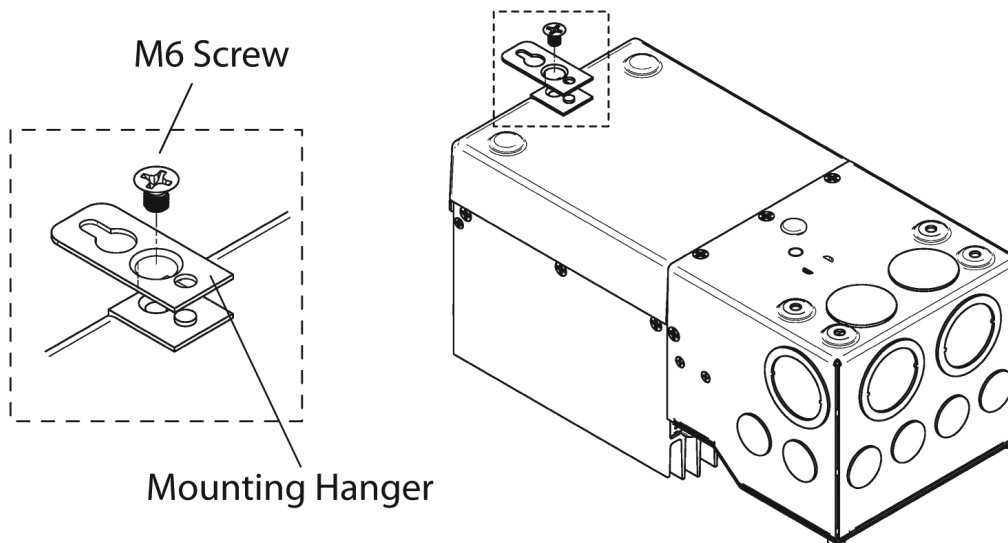
Abbildung 3-2: Befestigen der Montagehalterung
